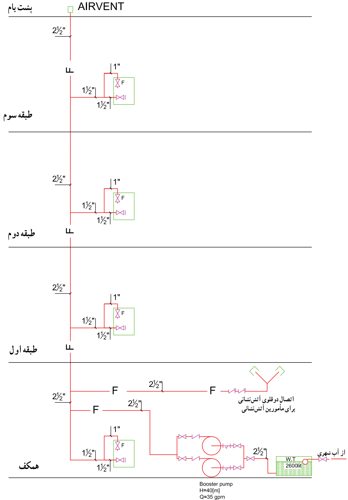
شکل ۲-۴ پ- رایزر دیگرام لوله‌کشی آب آتش‌نشانی
